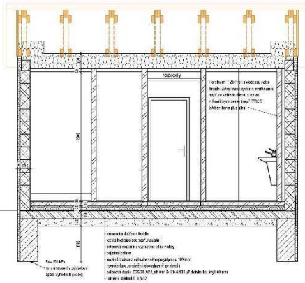
REZ PODÉLNÝ
